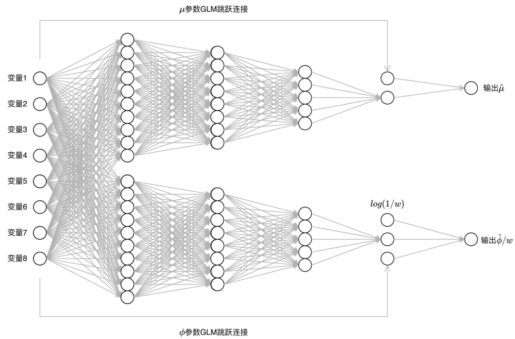
附图 1 双参数 Tweedie 组合神经网络的结构
